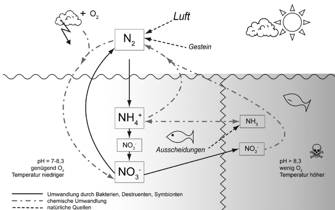
Abb. 1: Stickstoffkreislauf
