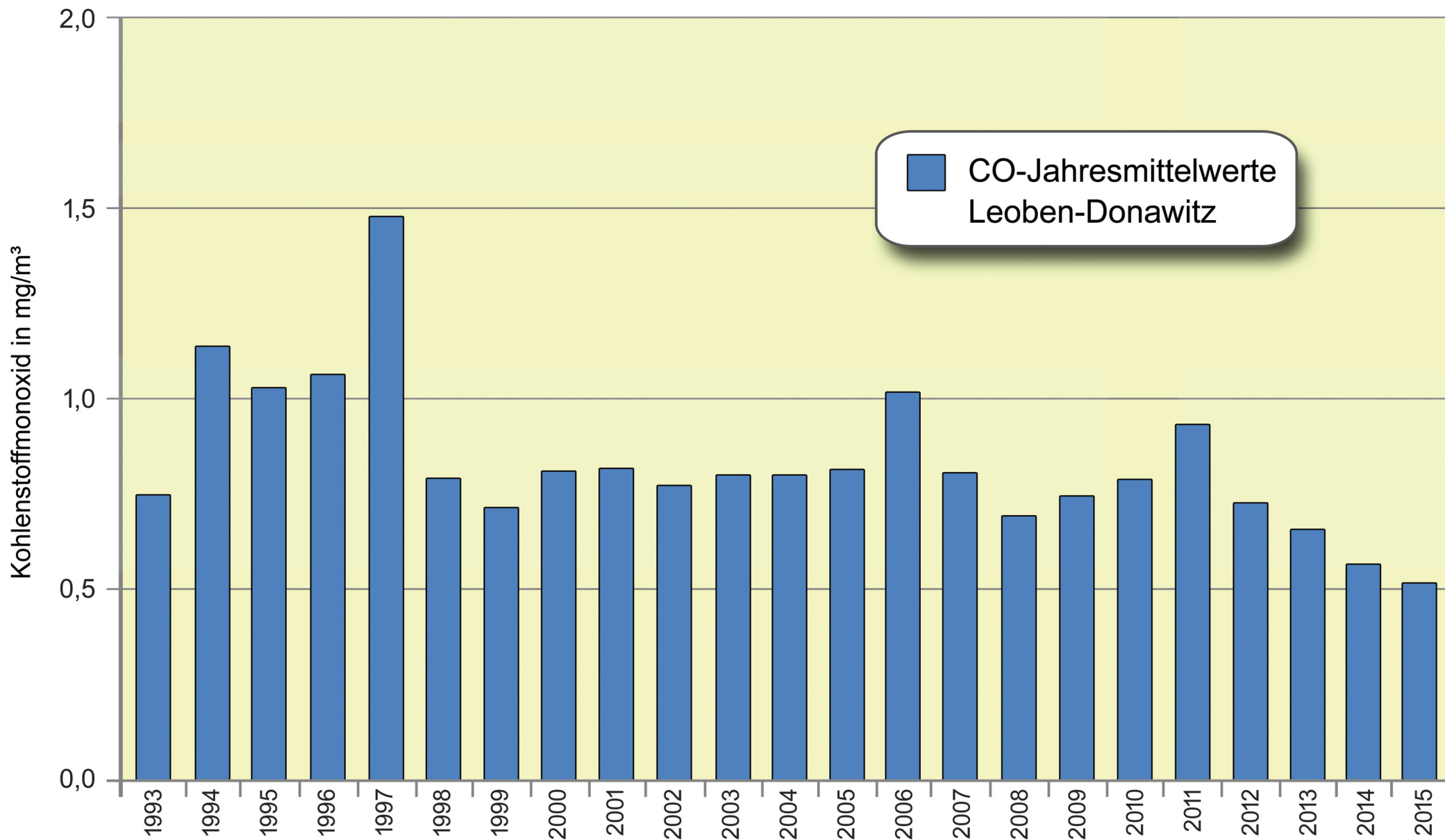
Abb. 74: CO-Jahresmittelwerte an der Station Leoben-Donawitz von 1993 bis 2015
