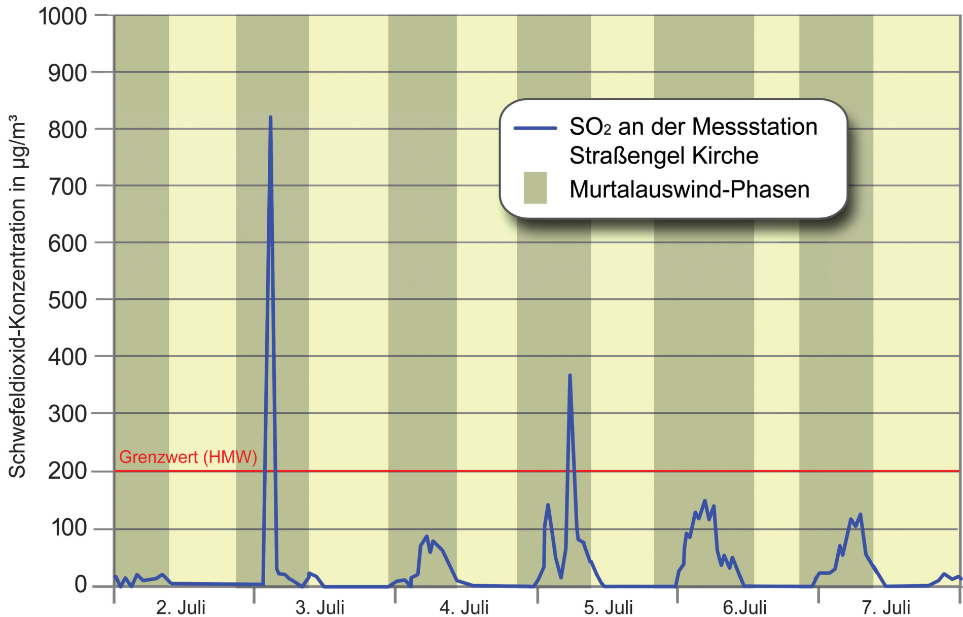
Abb. 69: Schwefeldioxidwerte an der Station Straßengel Kirche Anfang Juli 2015 zeigen den deutlichen Zusammenhang mit dem Talwindssystem.
