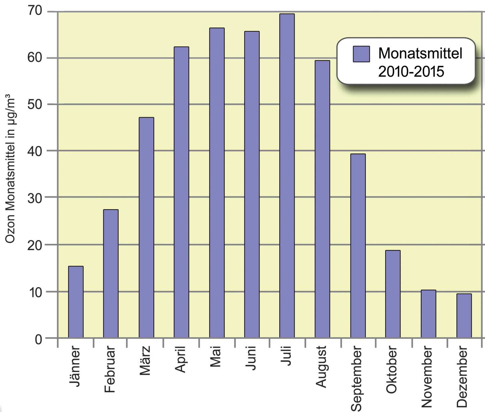
Abb. 62: Jahresgang der Ozon-Belastung an der Messstation Graz-Nord. Die Balken zeigen die durchschnittlichen Monatsmittelwerte über den Zeitraum 2010-2015.
