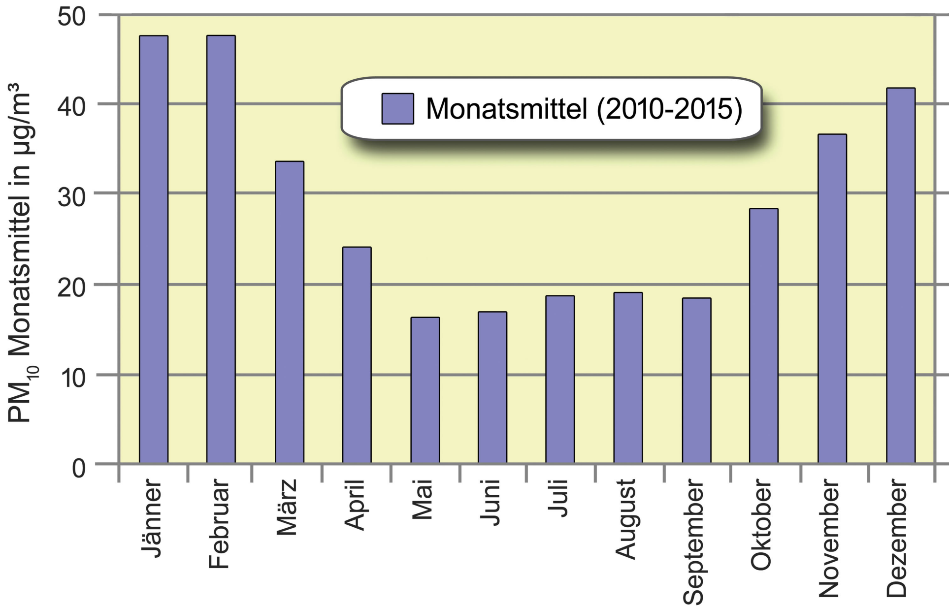
Abb. 49: Jahresgang der Feinstaub-Belastung an der Messstation Graz-Süd. Die Balken zeigen die durchschnittlichen Monatsmittelwerte über den Zeitraum 2010-2015
