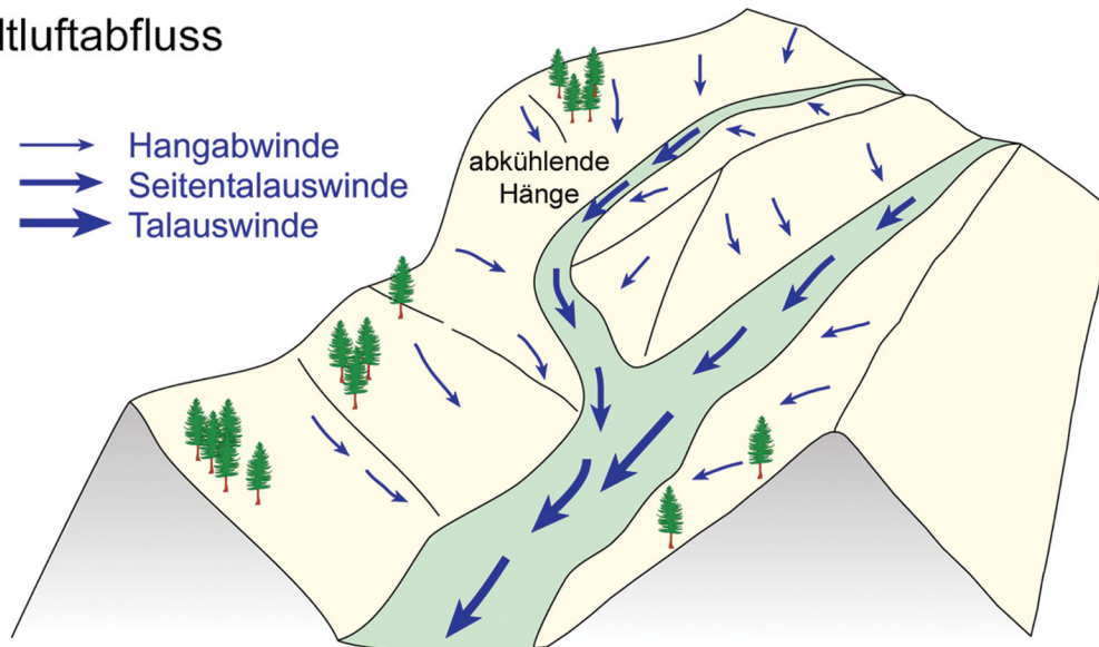
Tal mit Kaltluftabfluss
