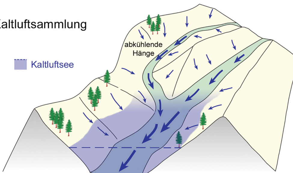
Tal mit Kaltluftansammlung
