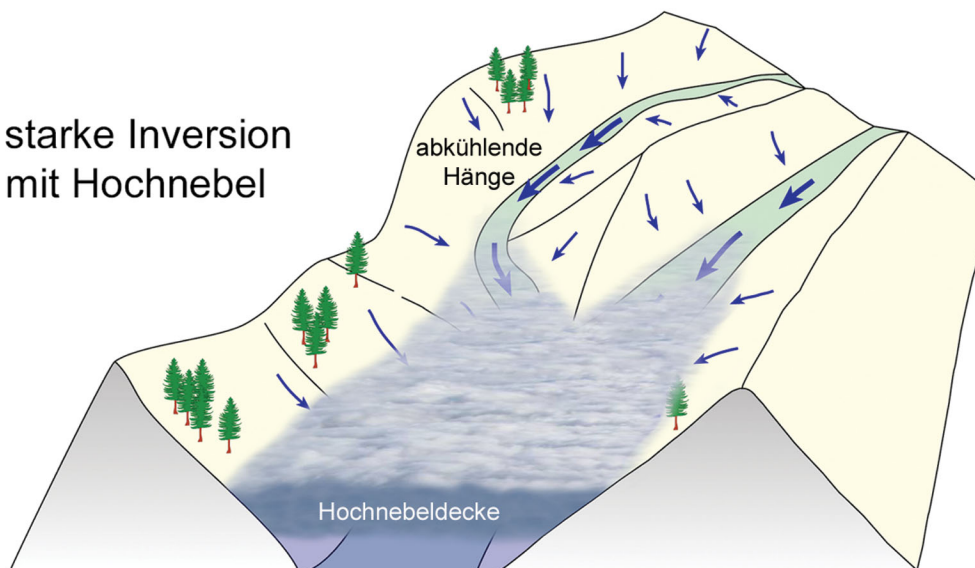
Tal mit Kaltluftsee und Inversion
