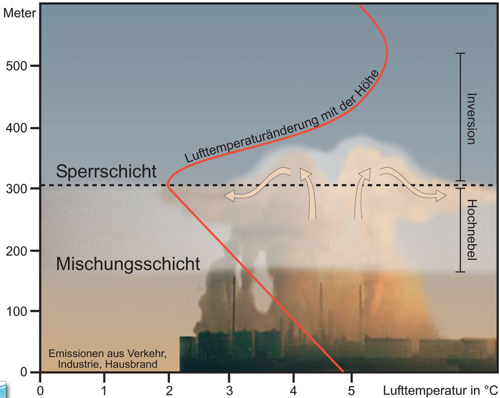
Abb. 33: Verhalten von Emissionen bei einer freien Inversion
