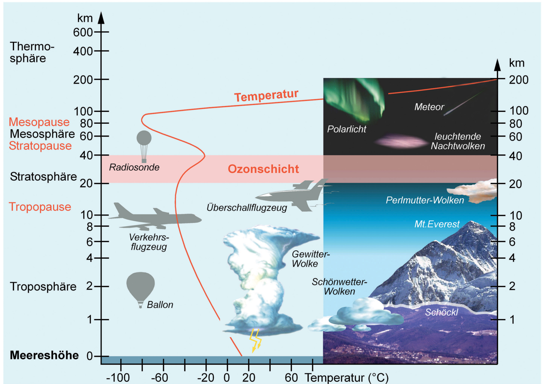
Abb. 10: Die Schichtung der Atmosphäre (logarithmische Höhenskala) in mittlerer geographischer Breite
