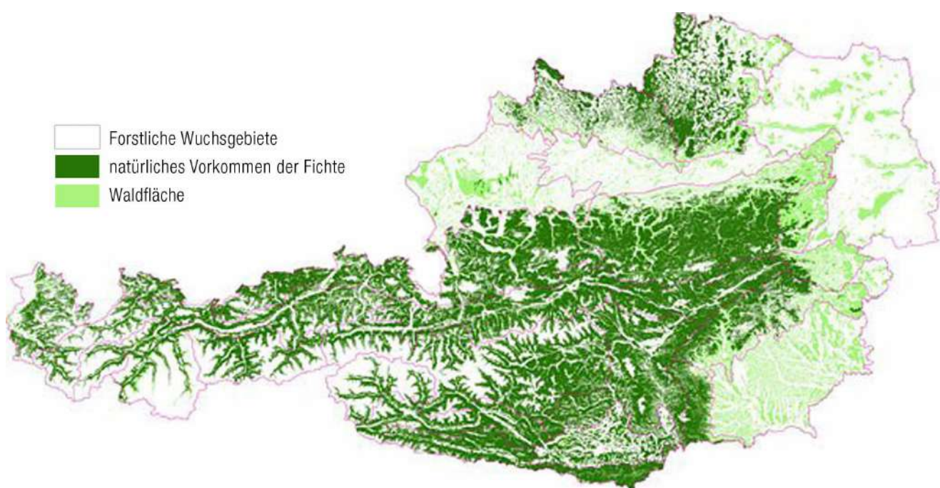
Abb. 14: Natürliche Verbreitung der Fichte vor der Klimaerwärmung; Büchsenmeister, R., 2013, BFW-Praxisinformation 31: 3 - 6
